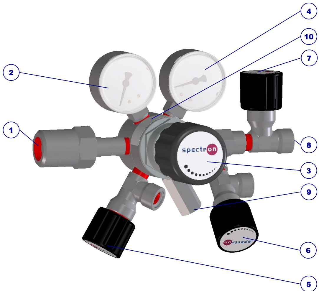
Abb. 1: Aufbau Druckregler FE51-SP
