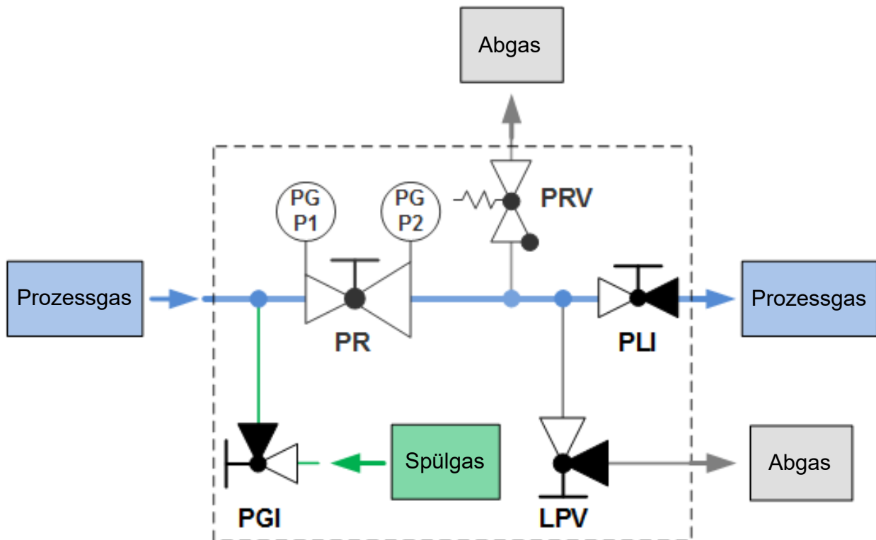
Abb. 2: Schema FE51-SP
