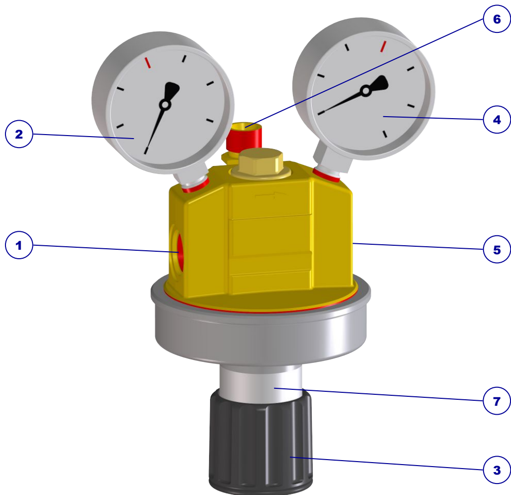
Abb. 1: Aufbau Druckregler U11
