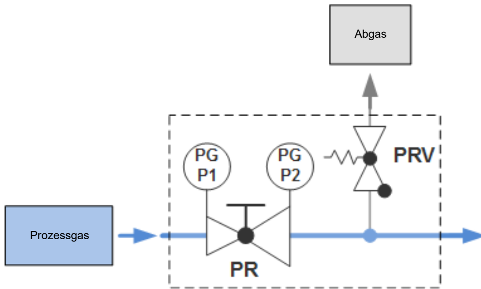
Abb. 2: Schema U11
