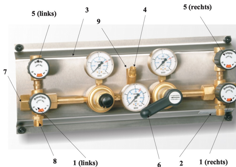
Afbeelding 2: CRS2000-2L beschrijving onderdelen
