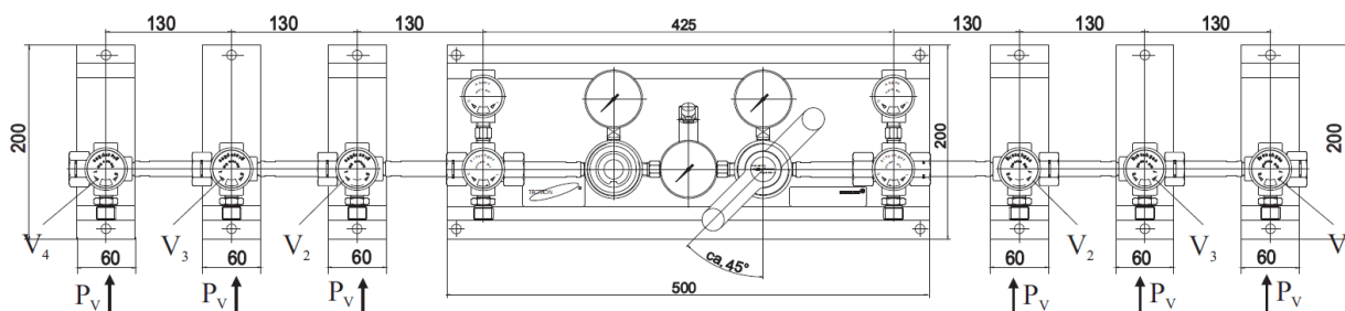
Afbeelding 3: CRS2000-2L met uitbreidingen tot 2x3
