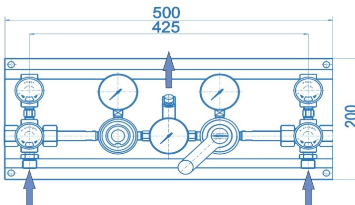
Afbeelding 1: CRS2000-2L-2x1 afmetingen
